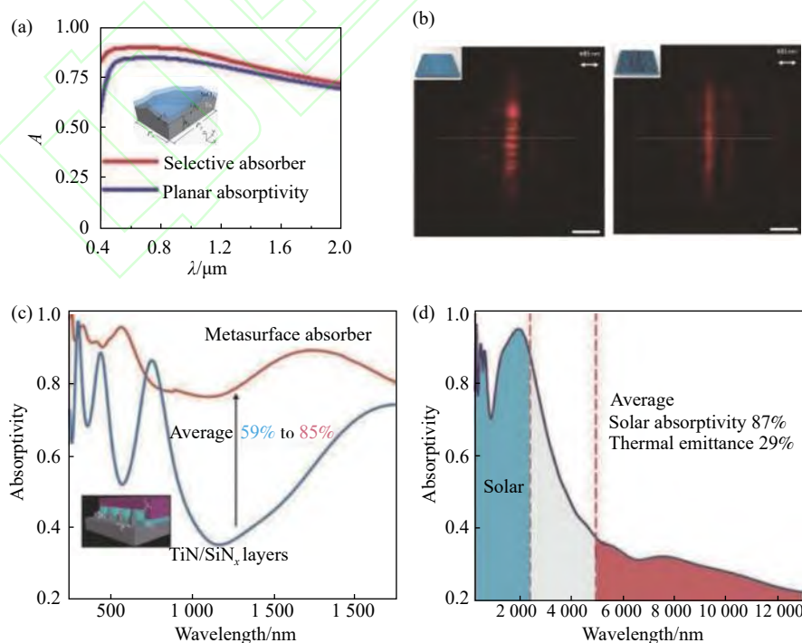
图 19 (a) SiO 2 -Ge-W 结构及其吸收谱图 [146] ; (b) 实验焦线强度的剖面图 [149] ; (c)-(d) SiN x -TiN-SiO 2 结构及吸收谱图 [150]
