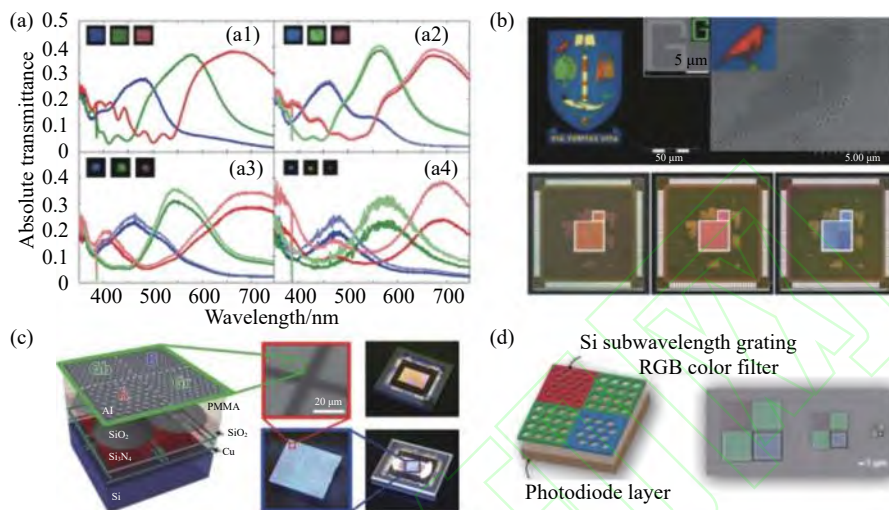
图 12 纳米孔阵列亚波长光栅滤光片。(a) 基于金属铝的纳米孔阵列滤光片, 尺寸边长分别为 (a1)10 \mu\text{m} , (a2)5 \mu\text{m} , (a3)2.4 \mu\text{m} , (a4)1.2 \mu\text{m} 的滤光片光谱 [87] ; (b) 纳米孔阵列形成的彩色徽标 [88] ; (c) 与 CMOS 图像传感器结合的纳米孔阵列滤光片 [89] ; (d) 基于硅材料亚波长光栅滤光片 [90]
