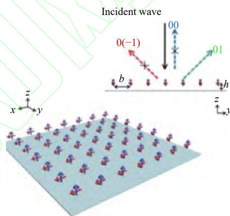
图 2 超构光栅的提出 [7]
