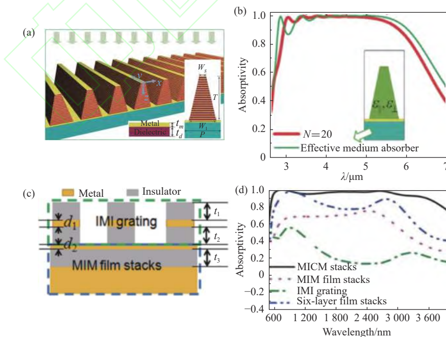
图 16 亚波长光栅(各向异性超材料薄膜)(a) 结构图及 (b) 吸收谱图 [118] ; (c) MICM 结构示意图; (d) 不同结构的吸收谱对比图 [119]
