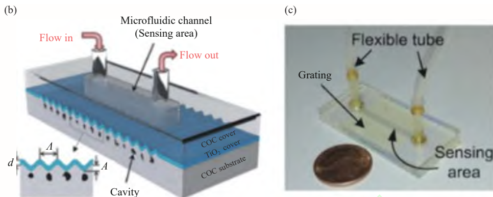
图 11 (a) 具有纳米级结构和逐点测量传感功能的微流控芯片示意图 [78] ; 一次性导模共振生物传感器芯片的 (b) 示意图和 (c) 其光学图像, 包括在环烯烃共聚物 (COC) 基板上的亚波长光栅 (一维 \text{TiO}_2 光栅) 结构和用于处理注射液的微流体模块 [80]
