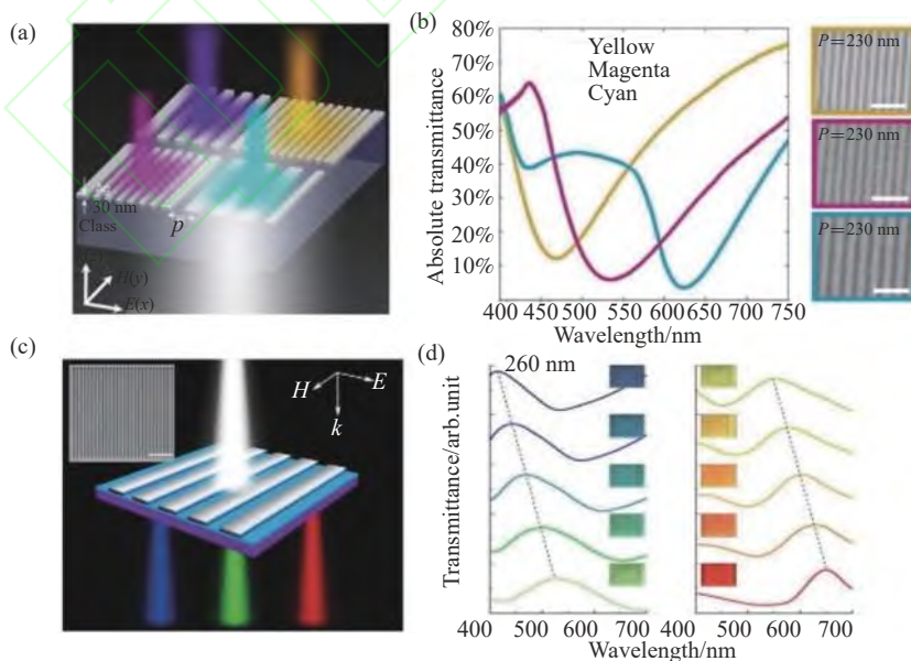
图 13 一维纳米光栅滤光片。超薄银等离激元纳米光栅滤光片 (a) 结构示意图和 (b) 光谱图 [98] ; (c) 纳米光栅滤光片结构示意图; (d) 颜色光谱与滤光片光栅周期之间的关系 [100]
