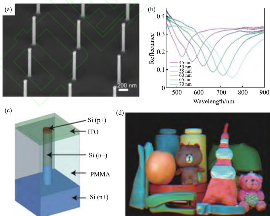
图 14 (a) 硅纳米线阵列扫描电子显微镜图。(b) 不同纳米线阵列的滤光片反射光谱 [105] ; (c) 垂直硅纳米线光电探测器的概念示意图; (d) 硅纳米线阵列拍摄测试对象的彩色图像 [106]
